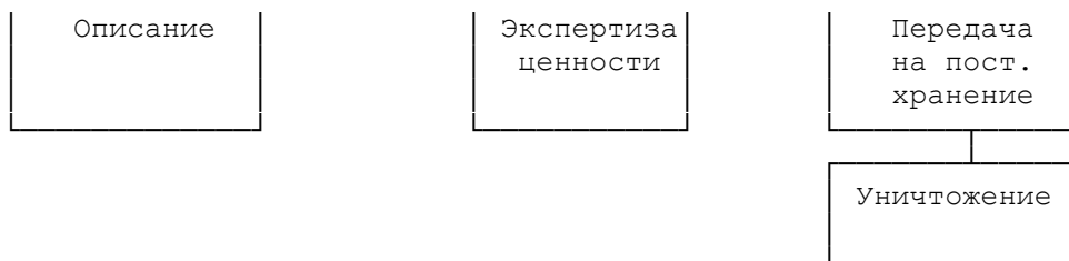
Схема 1
